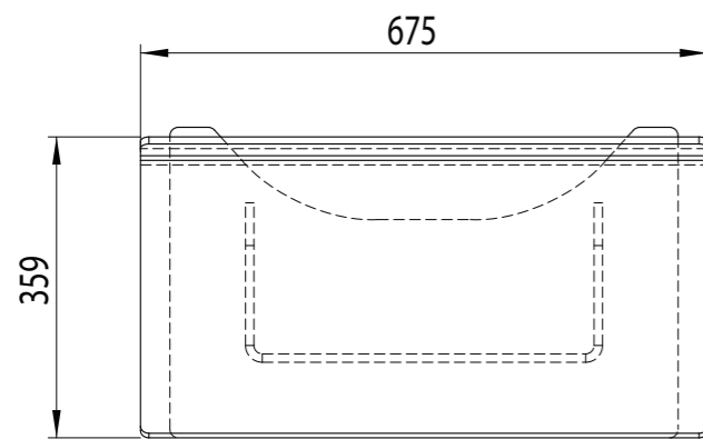
TOP ELEVATION SCALE: 1:10
