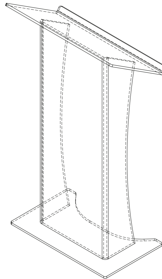
ISOMETRIC ELEVATION SCALE: 1:10
