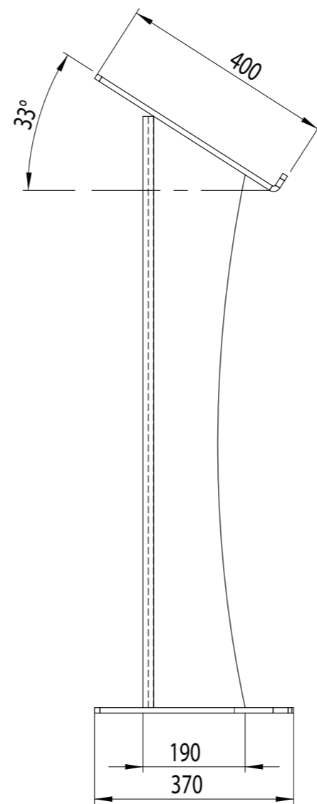
SIDE ELEVATION SCALE: 1:10
